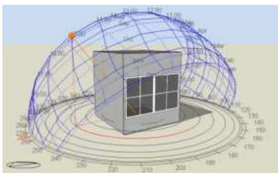
شکل 3 دیاگرام مسیر خورشیدی بر روی ساختمان طراحی شده
