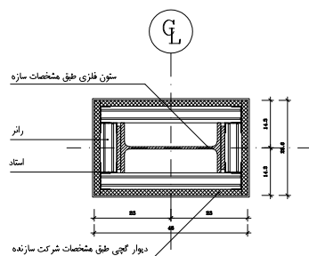
جزئیات پوششی ستون داخلی D-17 SC. 1:10
