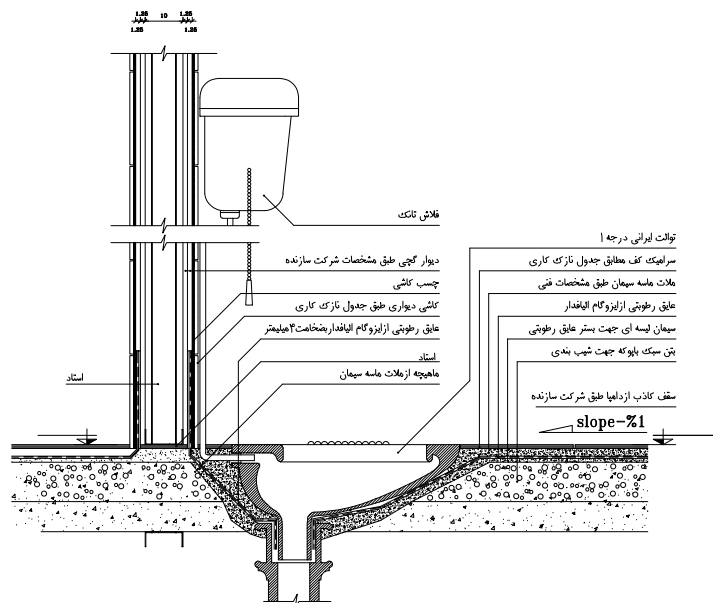
جزئیات اجرایی توالت ایرانی در طایفه اول
