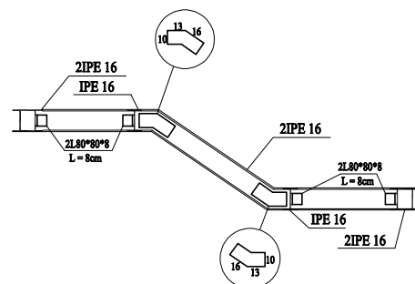
جزئیات اجرای رمپ پله
