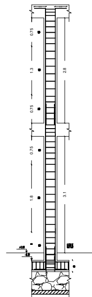
کلاف قائم ش 1:20
