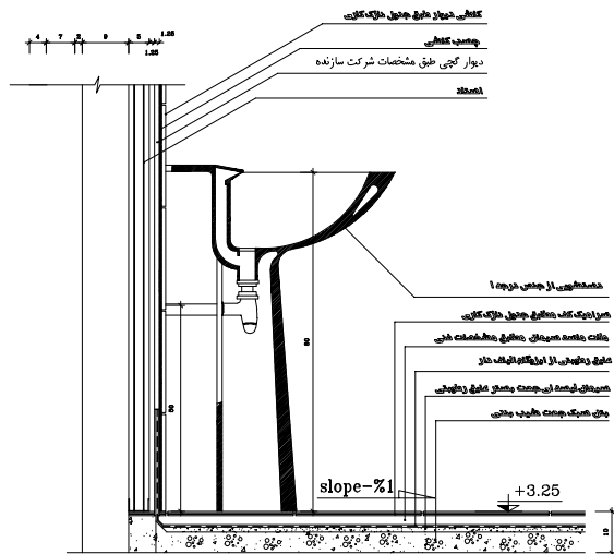
جزئیات اجرایی دستشویی در طبقه اول
