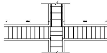
دیوار قائم ش 1:20
