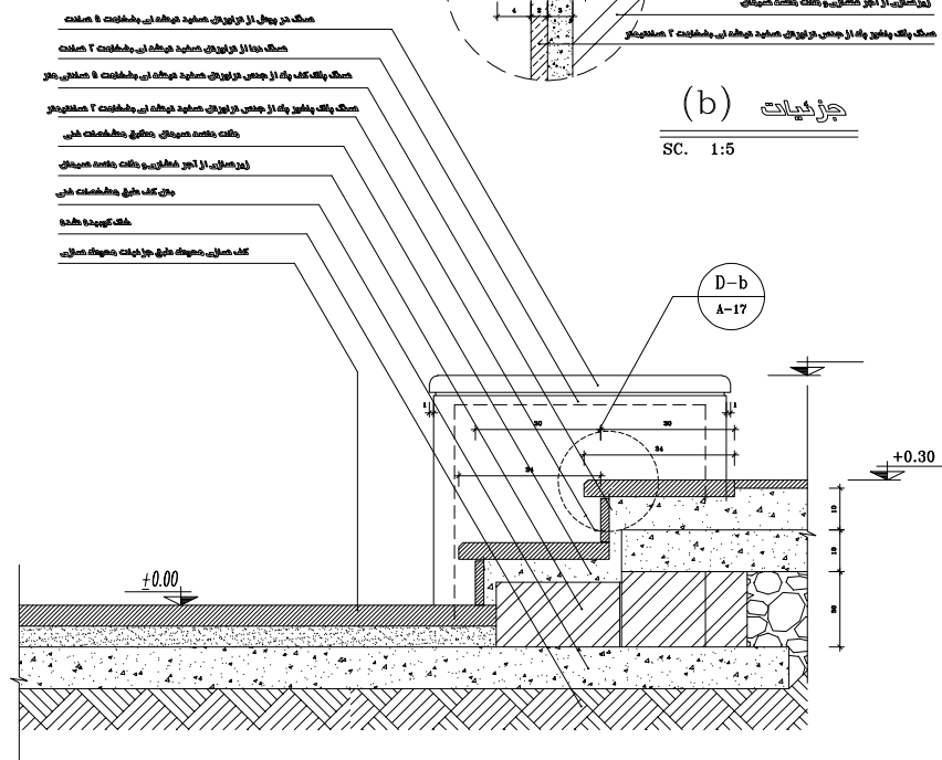
جزئیات اجرایی پله ورودی
