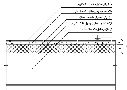
جزئیات گهسالی فضایی کشک در طبقات D-14 SC. 1:10
