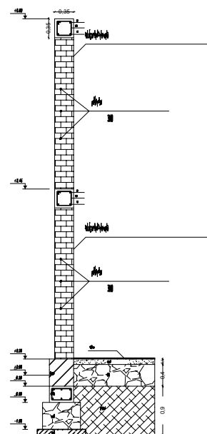
برش دیوار ش 1:20
