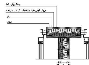
جزئیات گهسالی فضایی کشک در طبقات D-15 SC. 1:10
