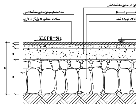
جزئیات گهسالی اطراف ساختمان D-12 SC. 1:10
