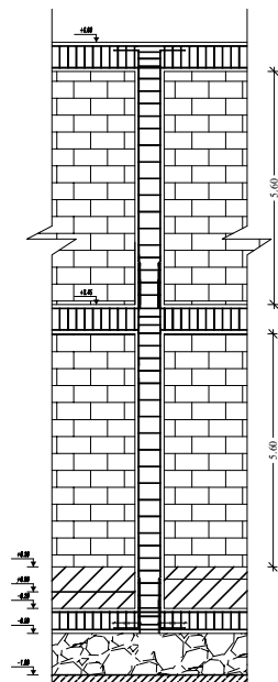
اجرای دیوار ش 1:20
