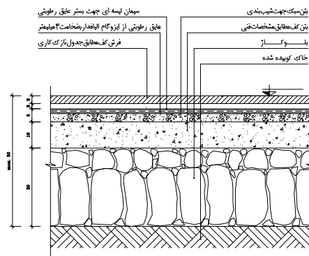
جزئیات گهسالی فضایی کشک در همگف D-10 SC. 1:10 (فضای سرویس بهداشتی و آشپزخانه)
