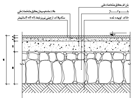
جزئیات گهسالی فضایی کشک در همگف D-9 SC. 1:10
