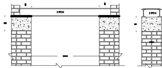
جزئیات اجرای نعل در گاهی در دهانه های 120 سانتی متری
