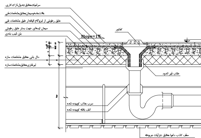
جزئیات کف نشو در طایفهات (سرویس های ما)
