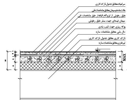
جزئیات گهسالی پانچ در راه پله D-11 SC. 1:10
