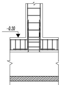
دیوار قائم ش 1:20
