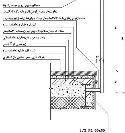
برش پله و اتصال خرده پله به آن (a-a)
