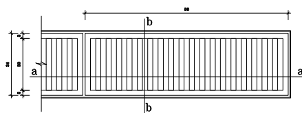
جزئیات اجرایی کانال عبور لوله های تأسیساتی
