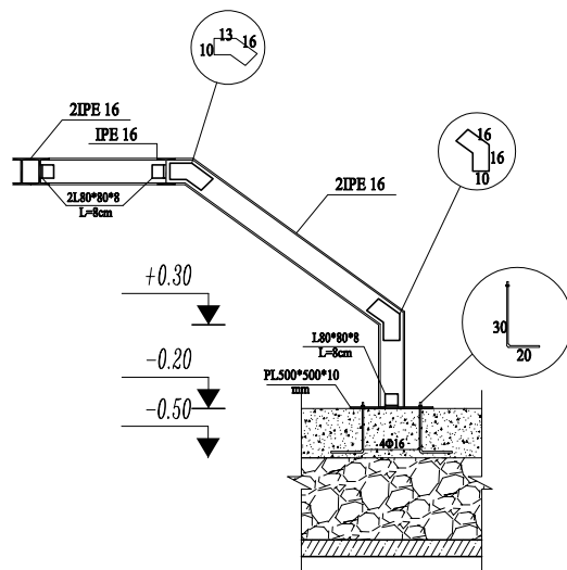
اتصال پله به فونداسیون
