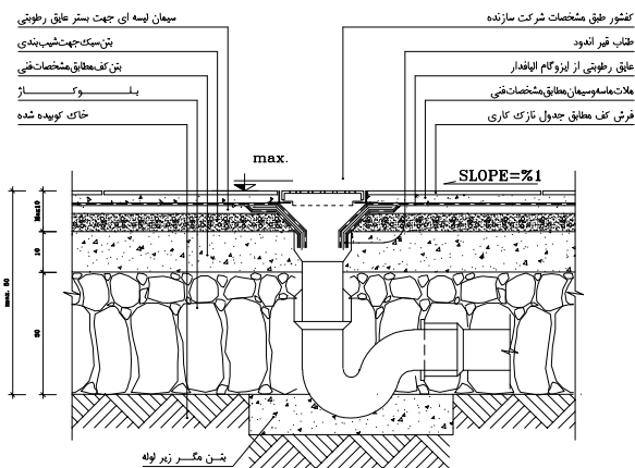
جزئیات اجرای کف نشوی آشپزخانه و سرویس در همگف D-13 SC. 1:10
