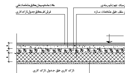
جزئیات گهسالی پانچ در راه پله D-11 SC. 1:10
